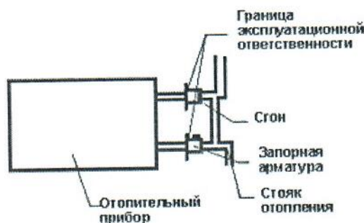
Рис.2 система отопления
