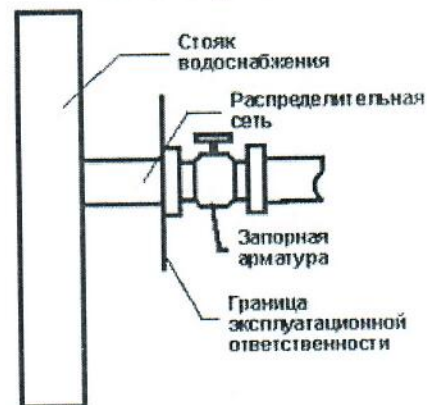
Рис.3 система водоснабжения
