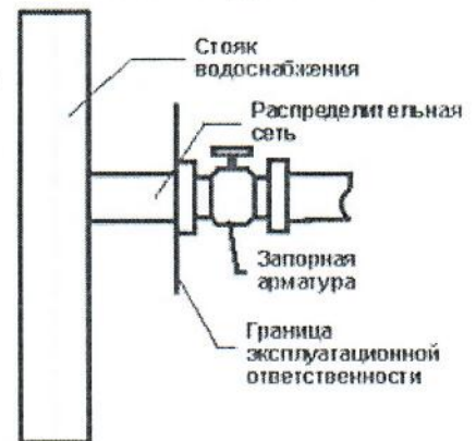
Рис.3 система водоснабжения
