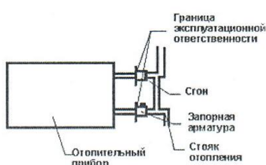
Рис.2 система отопления
