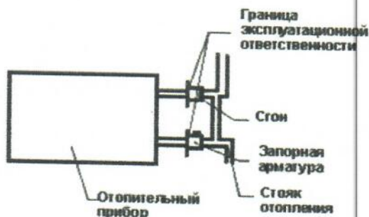
Рис.2 система отопления
