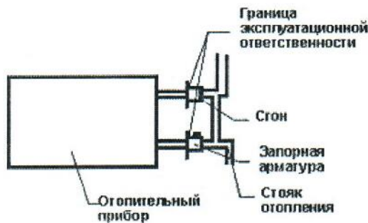
Рис.2 система отопления
