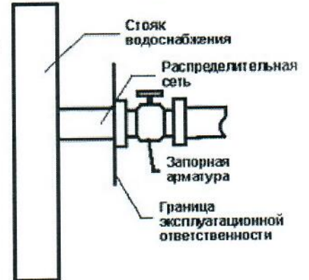
Рис.3 система водоснабжения
