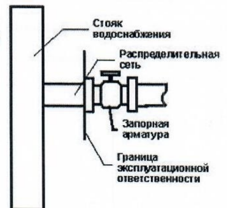
Рис.3 система водоснабжения
