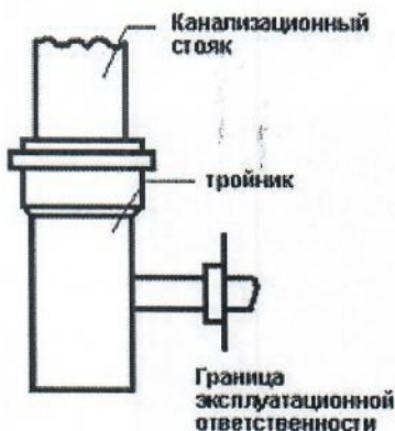
Рис.1 система водоотведения
