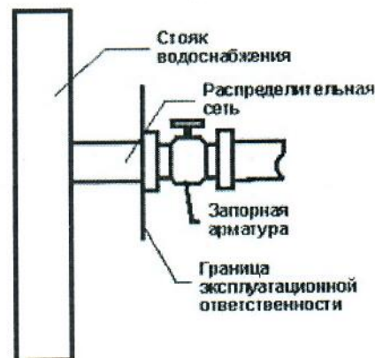
Рис.3 система водоснабжения
