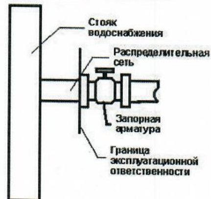
Рис.3 система водоснабжения
