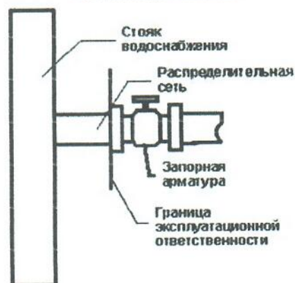
Рис. 3 система водоснабжения
