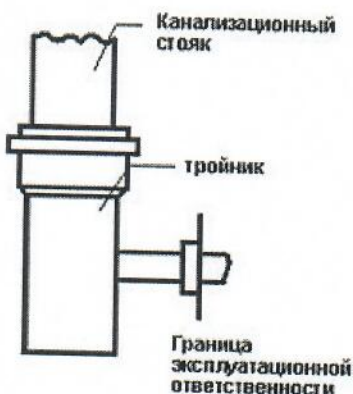
Рис.1 система водоотведения
