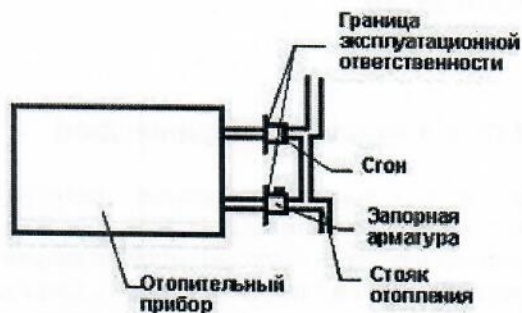
Рис.2 система отопления
