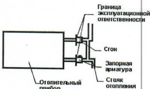
Рис.2 система отопления
