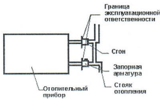
Рис.2 система отопления
